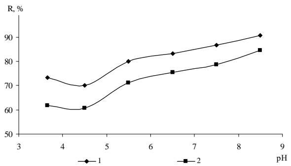
Рис. 5. Влияние pH на селективность (R) мембраны ОПМН-II при давлении 0,2 МПа по сульфатам (1), ионам жесткости (2) при степени отбора пермиата 10 %
