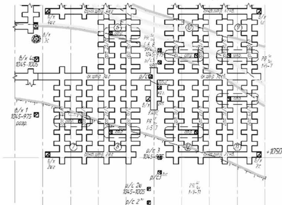
Рис. Вертикальные проекции (по буровым нишам и по отрезным щелям) и план горных работ блока 239 оси гор. 1035м
