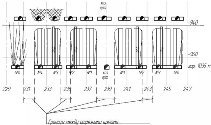
План гор. 1035м
