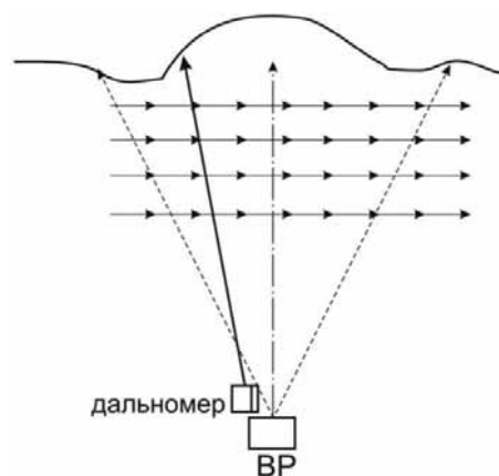
Рис. 3. Схема, иллюстрирующая принцип работы дальномера-видеорегистратора (BP)
