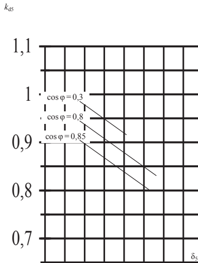
Рис. 2. Залежності підвищувального коефіцієнту k_{d5} від коефіцієнту \delta_5
