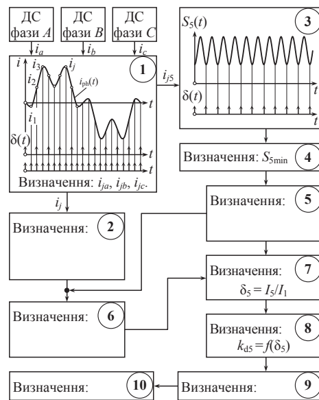
Рис. 4. Схема алгоритму спрацьовування мікропроцесорного пристрою захисту асинхронних електродвигунів від неупустимого перегріву обмоток
