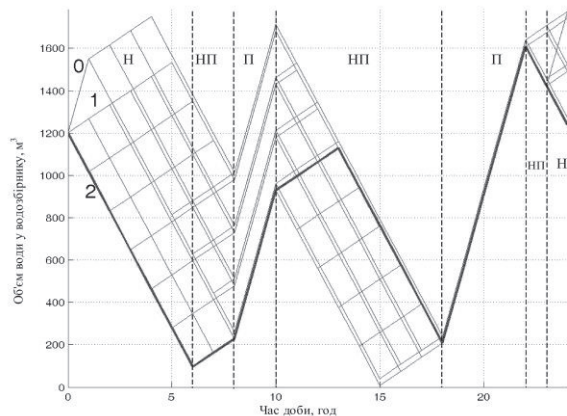
Рис. 3. Схема можливих режимів роботи ГВУ з двома насосами: 0, 1 і 2 – кількість одночасно працюючих насосів; Н, НП і П – відповідно, нічна, напівпікова та пікова зона доби
