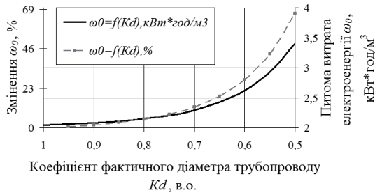
Рис. 1. Залежність питомої витрати електроенергії від зменшення внутрішнього діаметра трубопроводу
