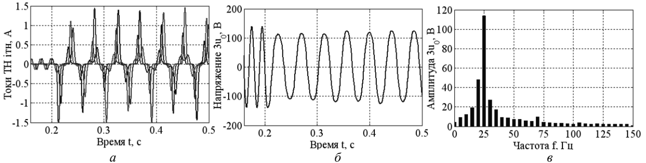
Рис. 1. Расчетные кривые токов в обмотке ВН трансформатора (а), напряжения 3u_0 (б), спектр напряжения 3u_0 (в) в режиме субгармонического феррорезонанса
