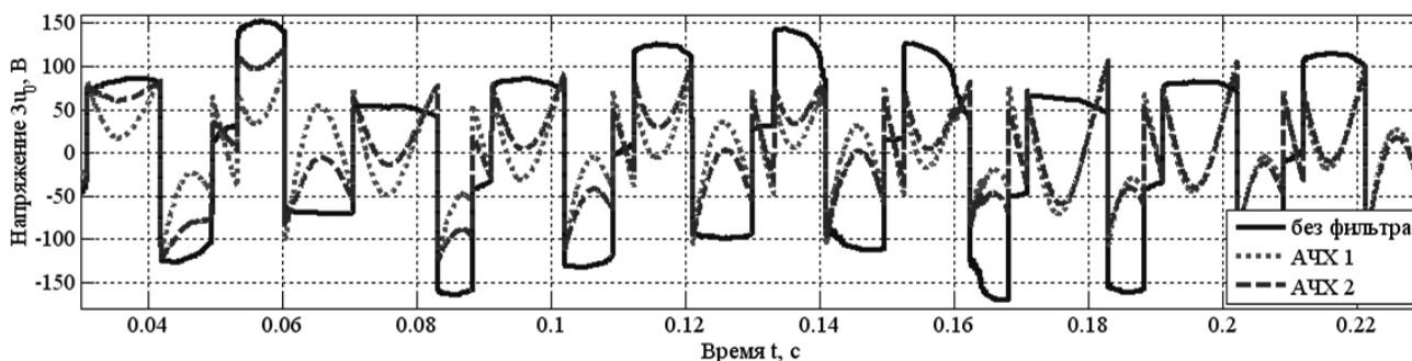
Рис. 8. Расчетные кривые напряжения 3u_0 в режиме ОДЗ без учета и с учетом режескторного фильтра
