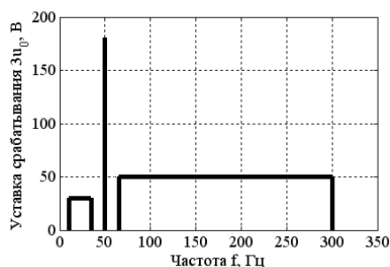
Рис. 3. Пороговые значения напряжения срабатывания напряжения 3u_0 при идентификации феррорезонанса
