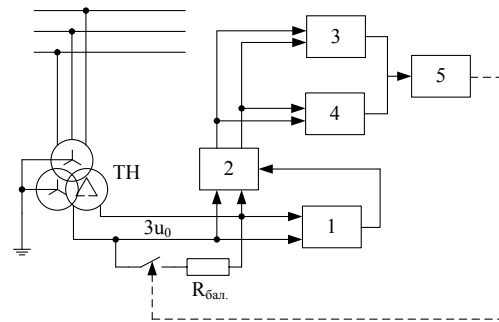
Рис. 2. Блок-схема разработанного устройства защиты от феррорезонанса: 1 – блок вычисления действующего значения напряжения 3u_0 ; 2 – блок сравнения действующего значения напряжения 3u_0 с уставкой; 3 – блок вычисления быстрого преобразования Фурье; 4 – блок отстройки от перемежающихся однофазных дуговых замыканий на землю; 5 – блок логического умножения; 3u_0 – мгновенное значение напряжения нулевой последовательности; ТН – трансформатор напряжения; R_{бал.} – балластное сопротивление
