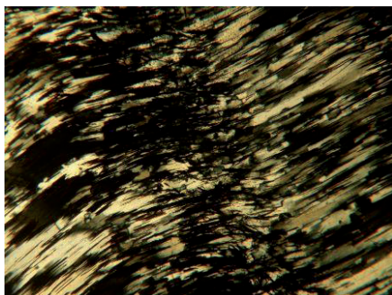
Рис. 5. Хвилястий вигин частково окварцованого паралельно-волокнистого агрегату кумінгтонітового азбесту, що надає мінливості, переливчастості забарвлення сірому соколиному оку. Прохідне світло; без аналізатора; збільшення 160\times
