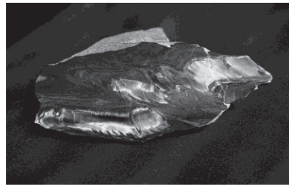
Рис. 8. Дислокований прожилок тигрового ока в магнетит-кумінгтонітовому кварциті сьомого сланцевого горизонту. Розмір зразка за максимальним виміром 11 см
