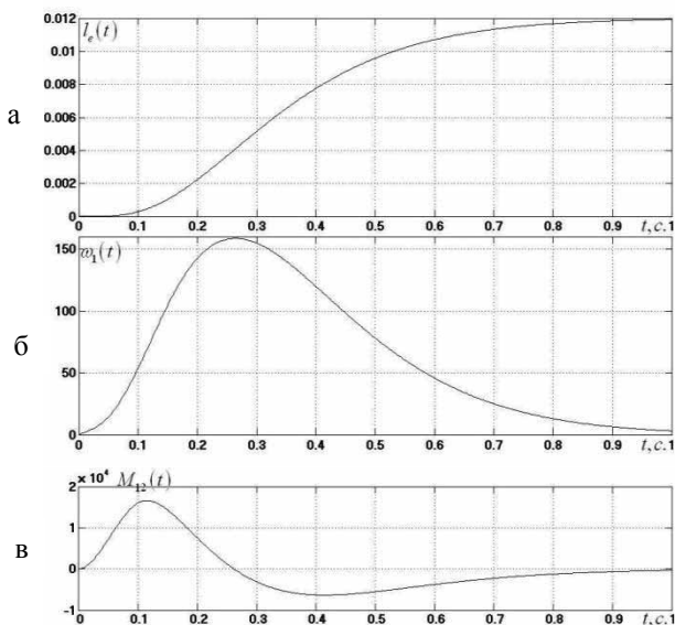
Рис. 5. Залежності траєкторій проміжних координат системи та сигналу керування від часу у випадку фазифікації лише l_e : умовні позначки див. рис. 3
