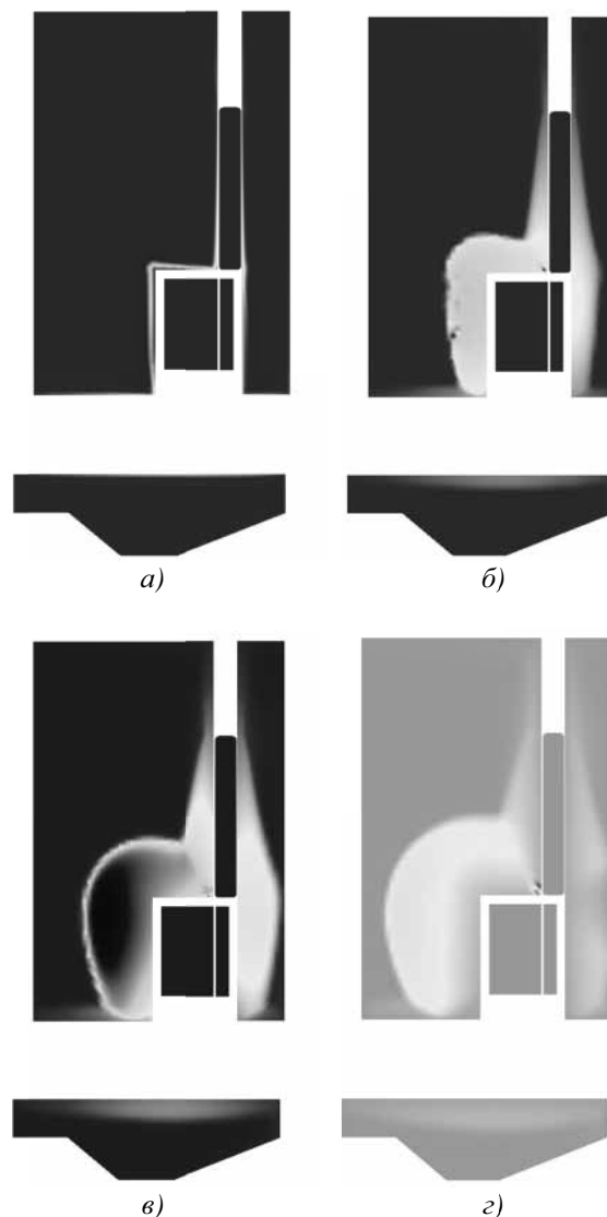
Рис. 6. Распределения вихревых токов в корпусе актуатора в моменты времени: а) 1 мс; б) 10 мс; в) 20 мс; з) 40 мс
